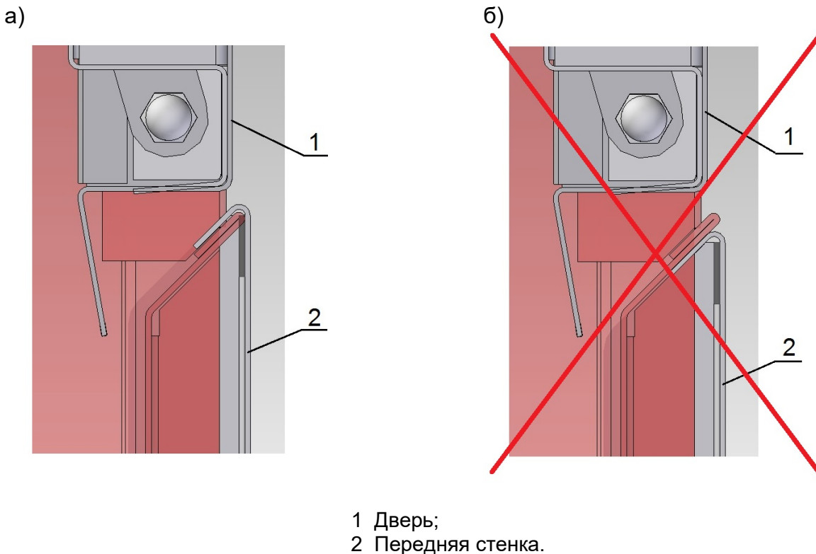
Рис. 6 Правильная (а) и неправильная (б) установка передней стенки
