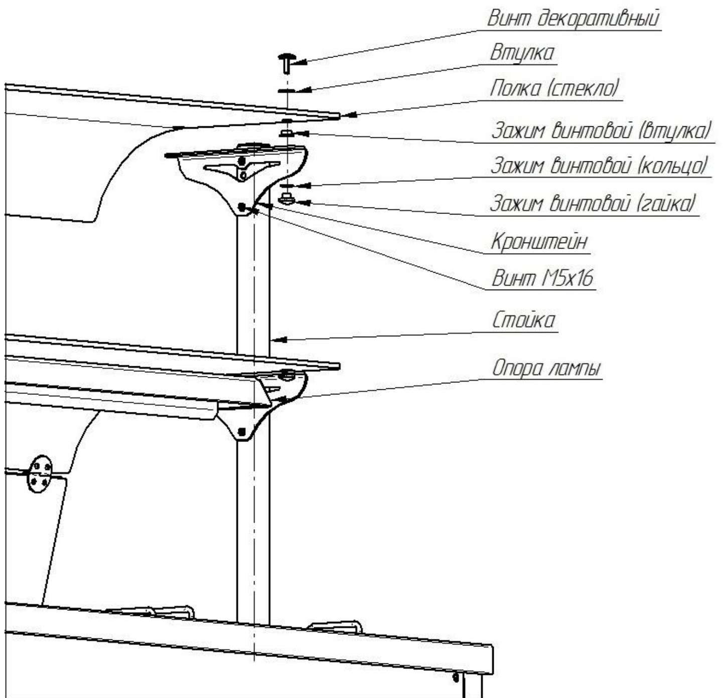
Рис.3 Сборка полок.
