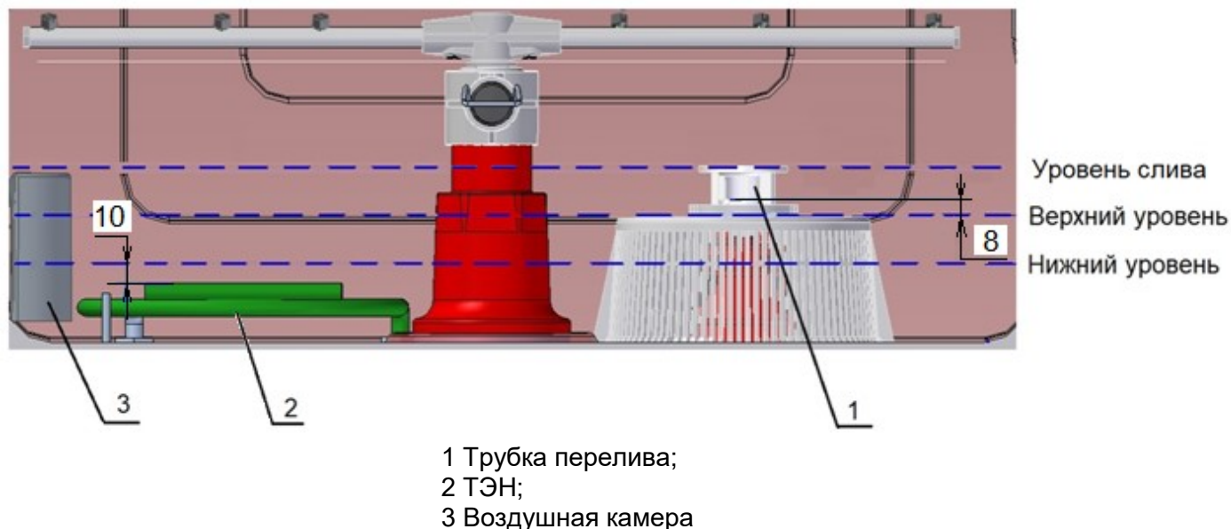
Рис. 4. Уровни воды в ванне
