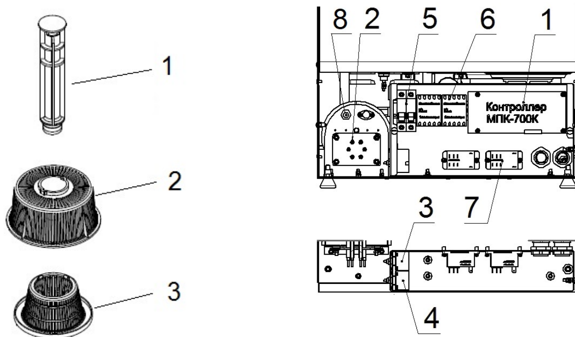
Виды спереди и сверху (передняя крышка снята)
