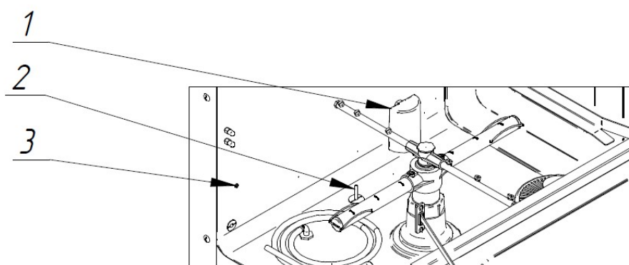
1 Воздушная камера; 2 Датчик температуры ванны; 3 Отверстие для подачи моющего средства
