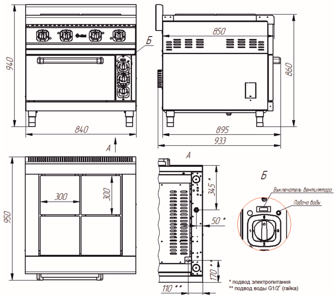
Рис. 15 Плита электрическая ЭПК-48ЖШ-K2/1
