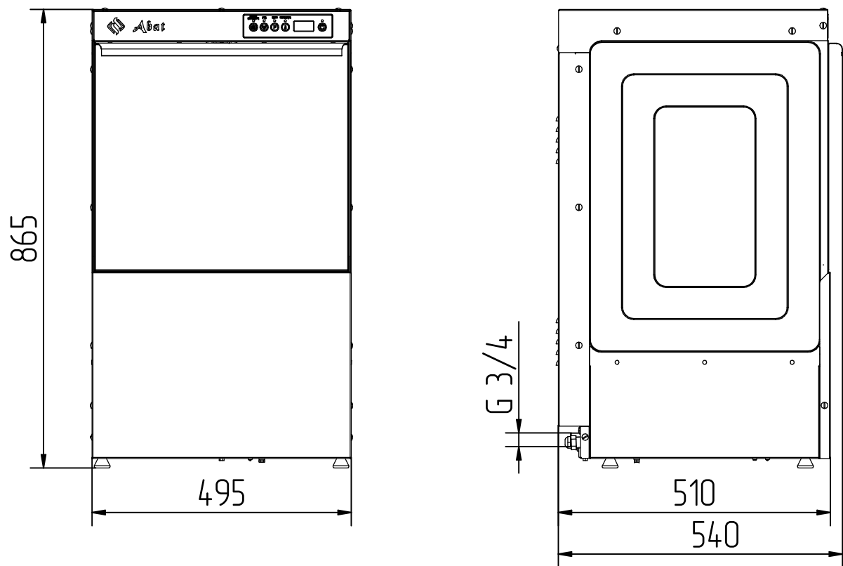
МПК-400Ф-01
