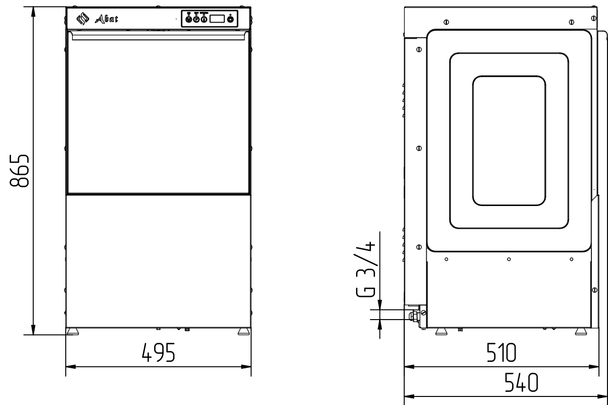
МПК-400Ф
